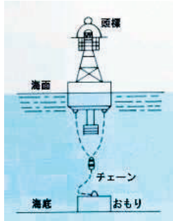
灯浮標の説明図
