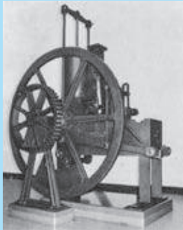
1812年イギリスで建造された汽船「コメット号」の蒸気機関 参考資料：小学館「船 航海のあゆみ」
