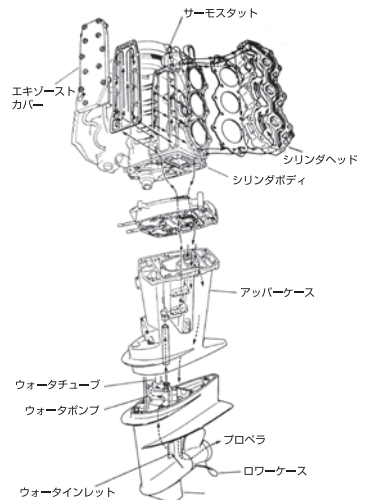
〈図1 冷却水経路〉
